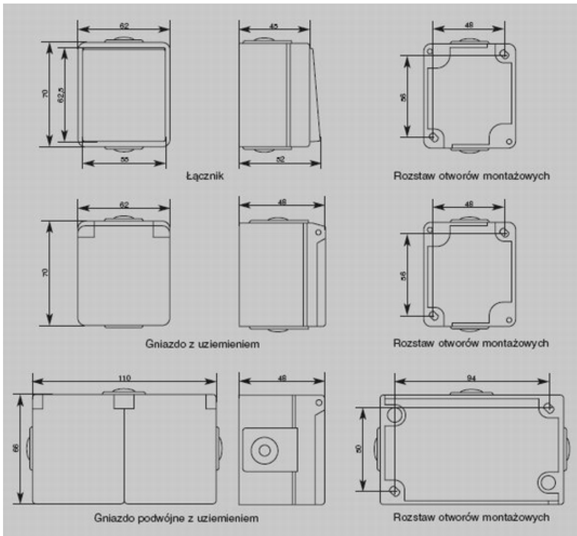
Wymiary gniazd i łączników hermetica
