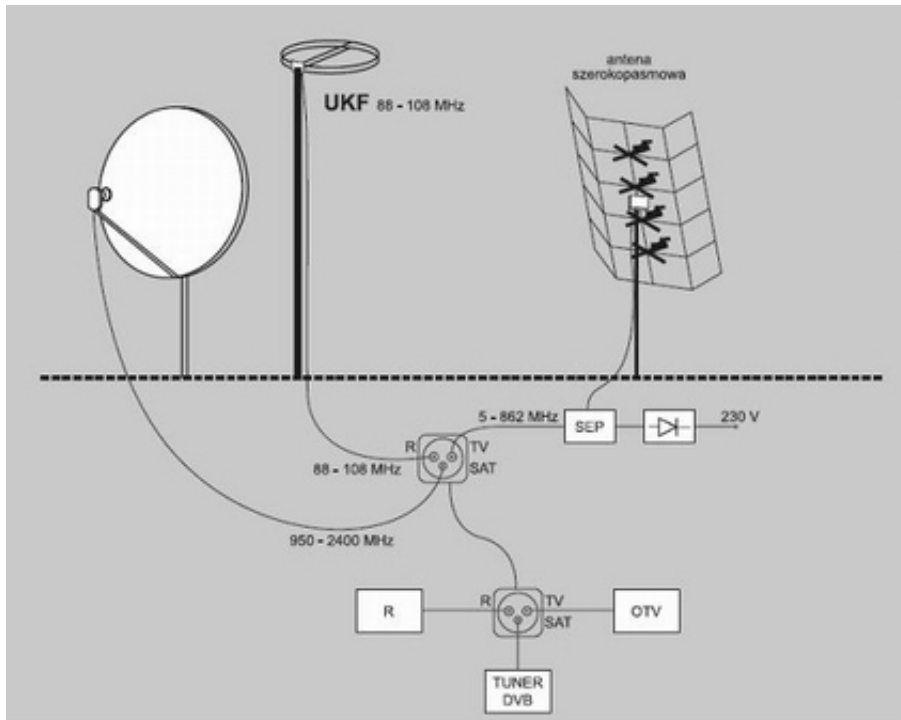
Indywidualna instalacja RTV SAT
